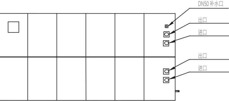
俯视图
