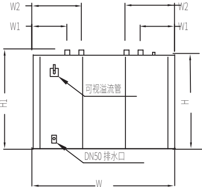
左视图
